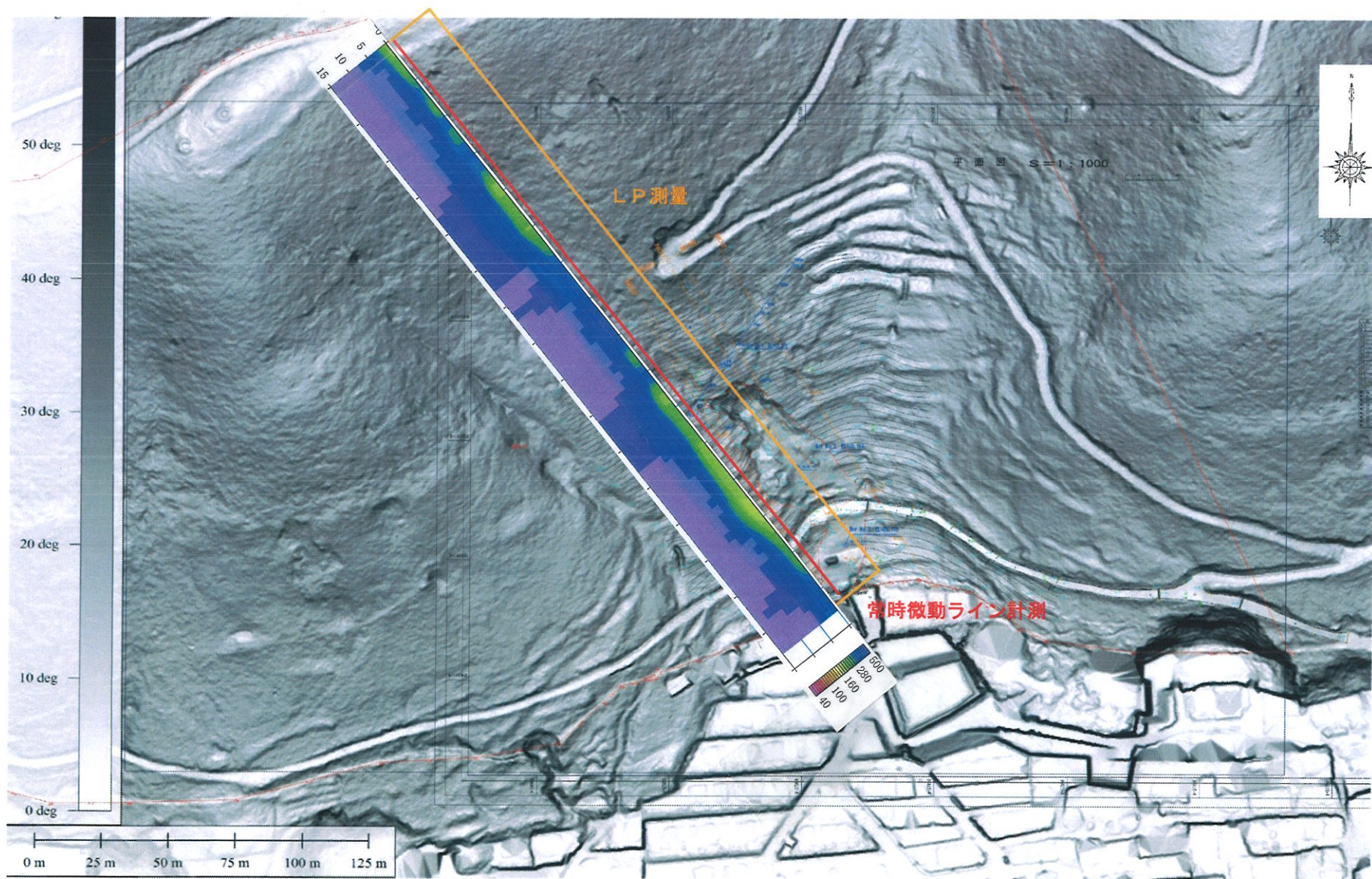
図-2 調査位置図 (※詳細は現地状況に応じ設定する)
